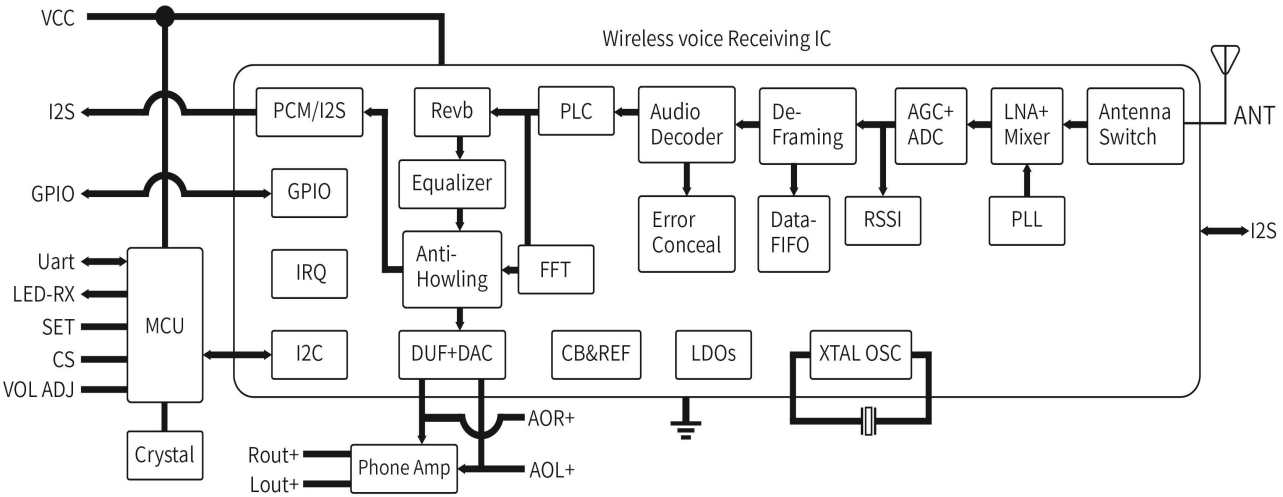
SA316-RX 方框图
