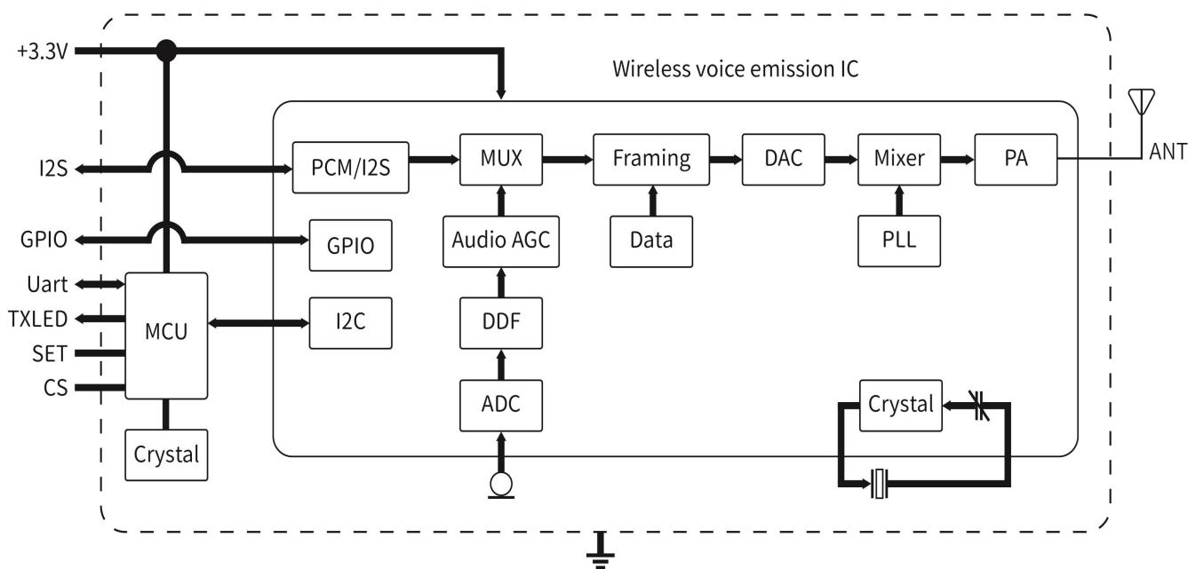
SA316S-TX 方框图
