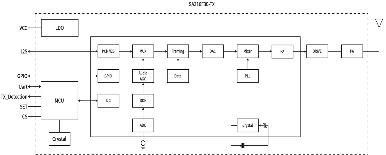
SA316F30-TX 方框图
